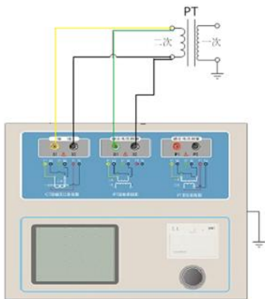
图 2-5 PT 直阻、励磁试验接线图
