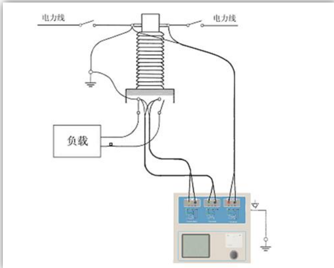
图 C-1 典型接线方式
