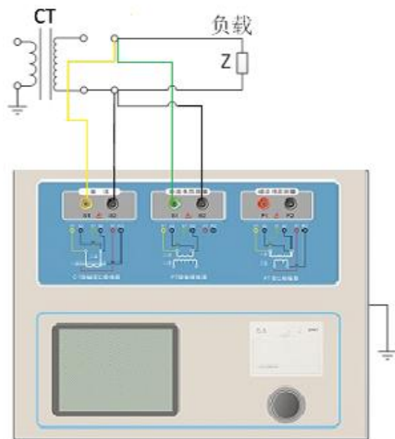
图 2-2 CT 二次负荷试验接线图
