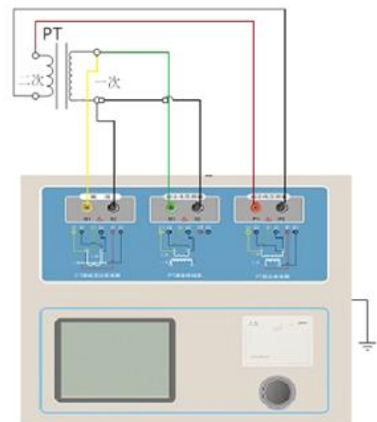
图 2-6 PT 变比极性接线图
